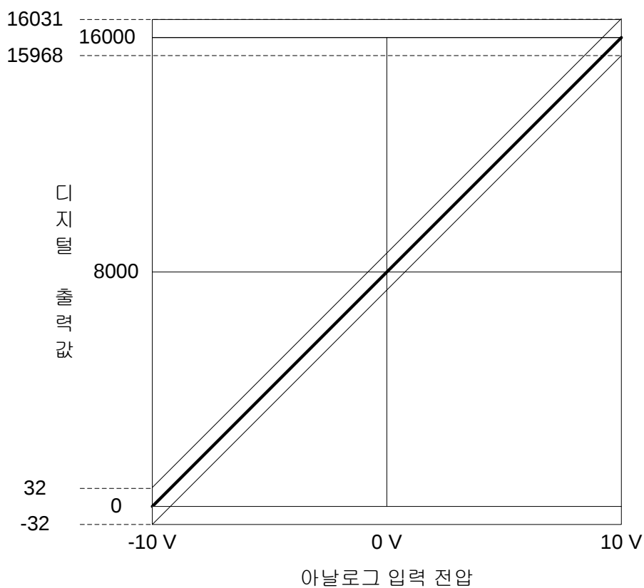
[그림 2.1] 정밀도( 25 \pm 5^\circ\text{C} 일 경우)
