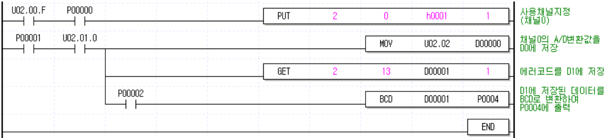
(b) PUT/GET 명령을 사용한 프로그램 예
