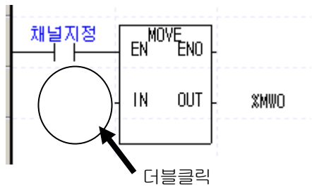
(a) 아래의 MOVE 평선을 이용하여 %MW0 로 A/D 변환 데이터를 읽어오는 부분에서 IN 앞 변수 부분을 더블 클릭하여 변수선택 창을 나타나게 합니다.
