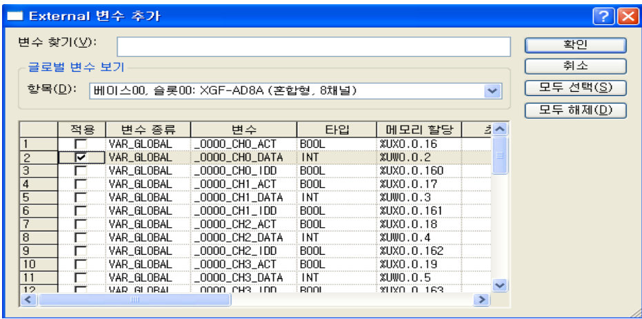
(d) 아래는 글로벌 변수 보기에서 “베이스00,슬롯00”의 디지털 입력값 (_0000_CH0_DATA)을 선택한 예 입니다.
