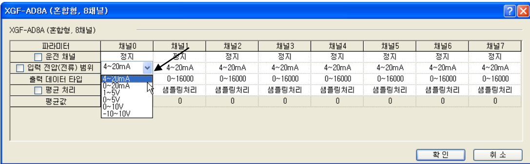
(b) 입력 범위: 사용하고자 하는 아날로그 입력 전압 또는 전류의 범위를 선택합니다. 아날로그 입력 모듈에서는 2가지 전류 입력범위를, 4가지 전압 입력 범위를 제공합니다.
