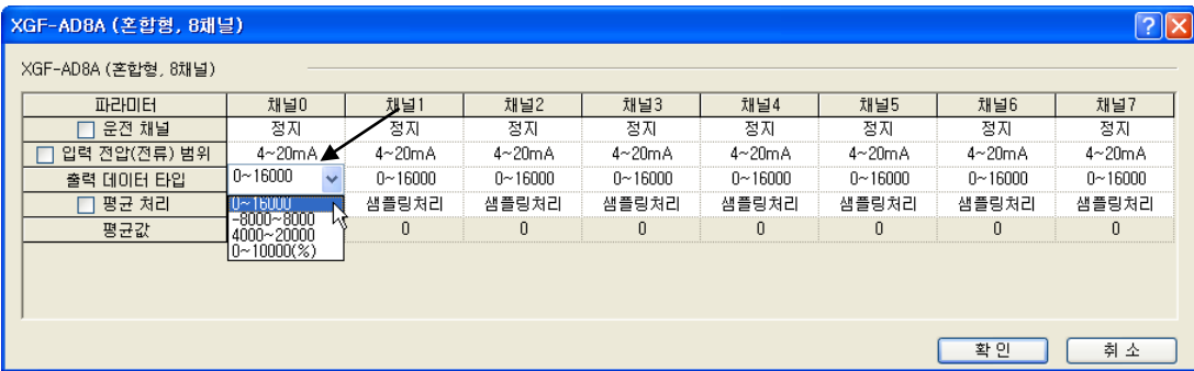
(c) 출력 데이터 타입: 출력 데이터 타입을 선택합니다. 선택할 수 있는 범위는 총 4가지입니다.
