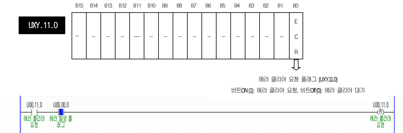
[그림 5. 1] 에러 클리어 요청 플래그 사용 방법
