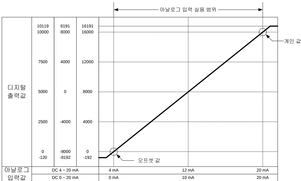
전류입력
